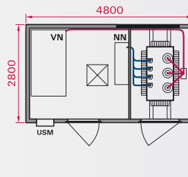
PŮDORYS
