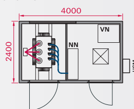
PŮDORYS
