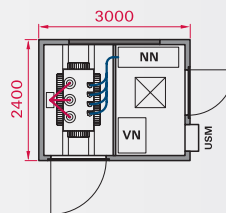
PŮDORYS
