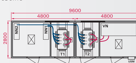
PŮDORYS
