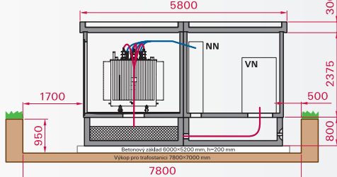
NÁRYS
