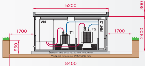
NÁRYS
