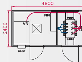
PŮDORYS
