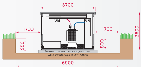
NÁRYS
