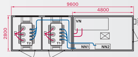
PŮDORYS
