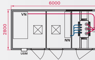
PŮDORYS
