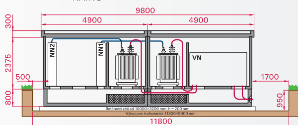
NÁRYS
