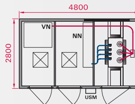
PŮDORYS
