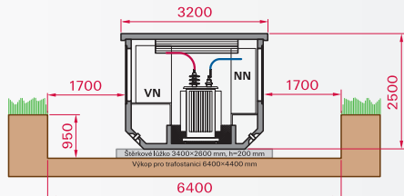
NÁRYS
