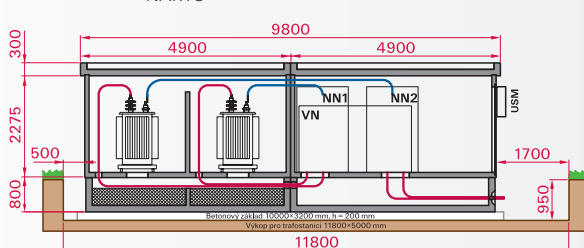
NÁRYS
